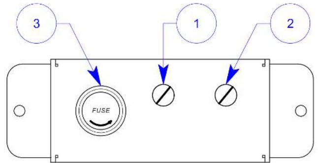
Рис. Блок настройки электрогенератора
